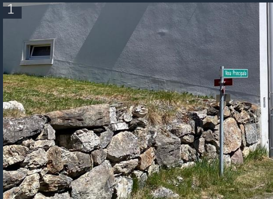
Bruchstein Stützmauer. Quelle: professor voser.
