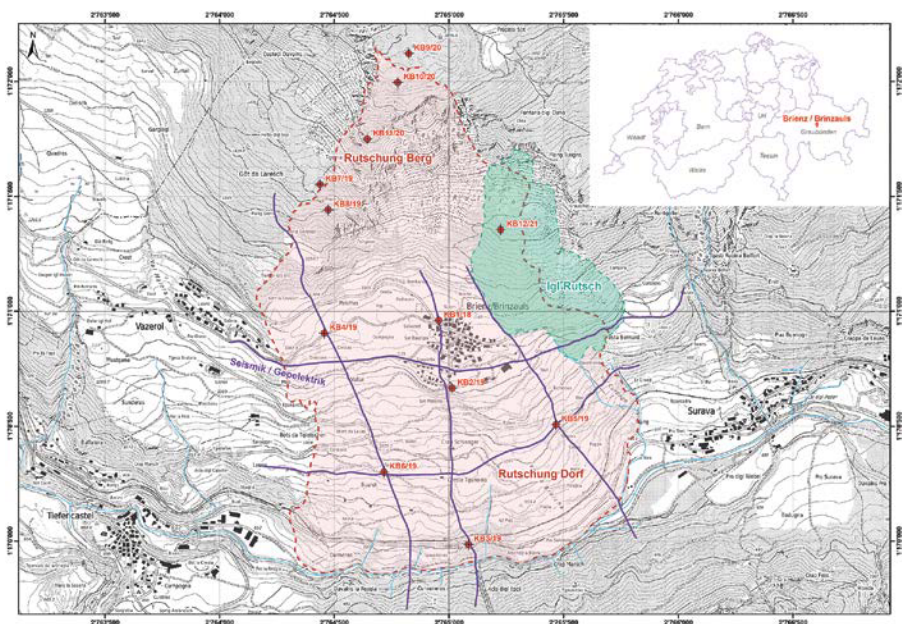
Abb. 1: Situation mit der Umrandung der Rutschung Brienz/Brinzauls, den Bohrstandorten und den Profilinien Seismik/ Geoelektrik. (Darstellung: zVg BTG AG)
