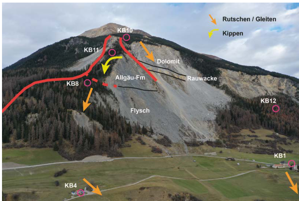
Abb. 4: Ansicht der Rutschung Brienz/Brinzauls mit den festgestellten Bewegungsmechanismen. (Darstellung: BTG AG)
