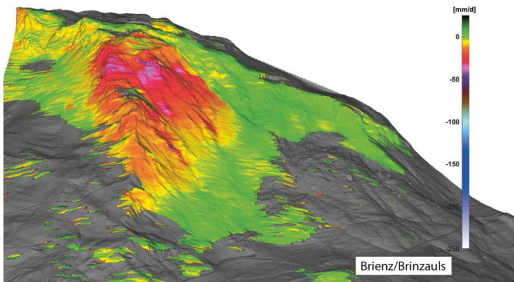
Abb. 3: Interferometrisches Radarbild der Rutschung Berg vom 11.8.2021, 12.01 Uhr. Die schnellen Bereiche «Insel» und «West» der Rutschung Berg sind in pink und rot deutlich erkennbar. Demgegenüber ist der Osten, in grün, stabil. Die stabilen Bereiche werden bei der Bildanalyse bewusst zum Abgleich verwendet.
