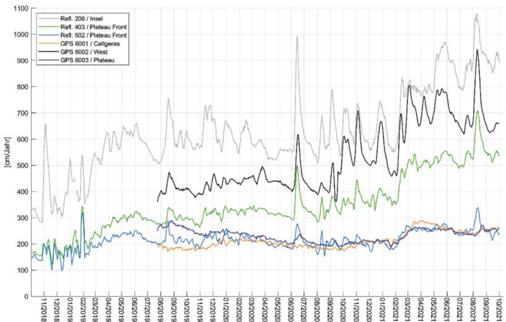
Abb. 4: Horizontalgeschwindigkeiten ausgewählter Messpunkte der Rutschung Berg (cm/Jahr).
