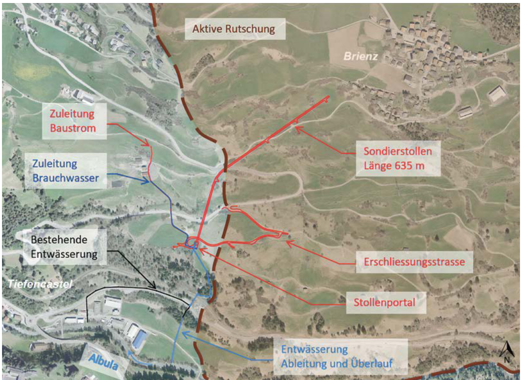
Situation Sondierstollen mit Erschliessungen.
