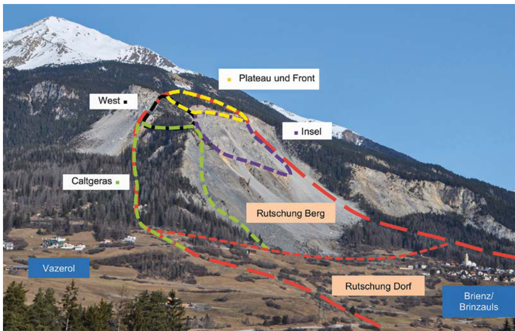
Abb. 1: Die Grossrutschung Brienz/Brinzauls wird in zwei Teilrutschungen und mehrere Einzelteile aufgeteilt. In diesem Zusammenhang werden verschiedene Ereignisszenarien abgeschätzt. (Illustration: CSD INGENIEURE AG)
