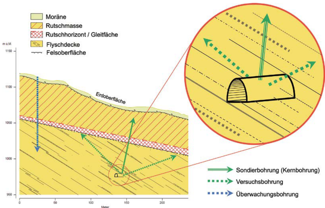
Der Sondierstollen im Schema: Einfach verständliche Grafiken und Bilder sind zentrale Elemente der Informationsvermittlung.
