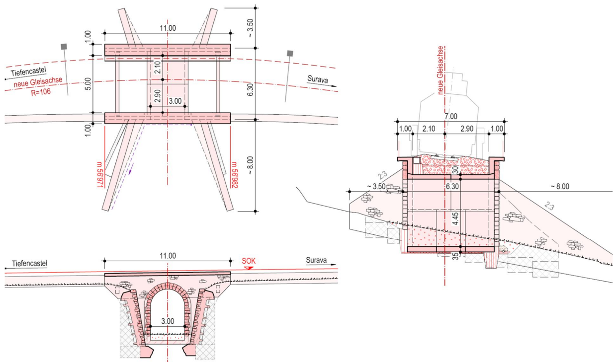
Abb. 2: Katasterplan neue Wegunterführung km 56.971
